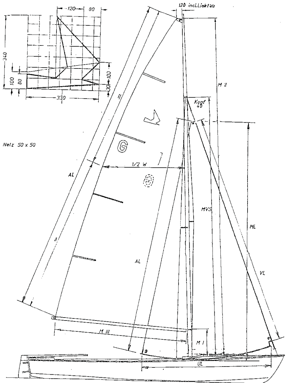
SCHWERT - ZUGVOGEL Segelriss M 1:50
